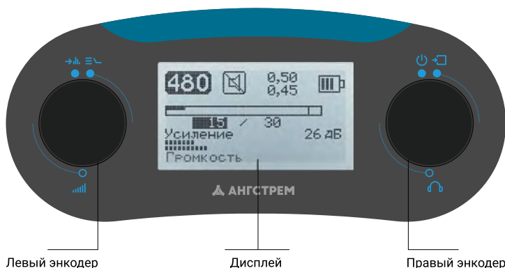
Рисунок 1 – Передняя панель приемника
