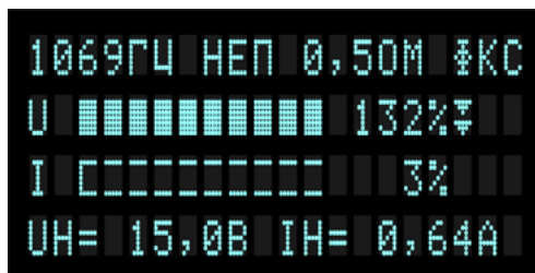
Рисунок 6.1 – Режим ограничения по напряжению (▼)
