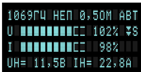
Рисунок 6.2 – Режим ограничения по мощности (▼S)
