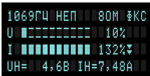
Рисунок 6.3 – Режим ограничения по току (▼)
