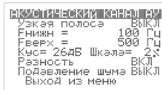
Рисунок 10 – Экран меню канала «АУ»
