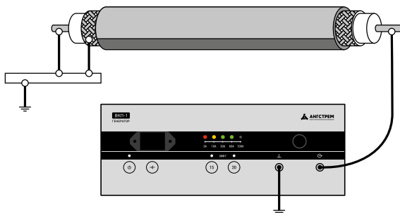
Рисунок 3 – Подключение генератора к однофазному экранированному кабелю
