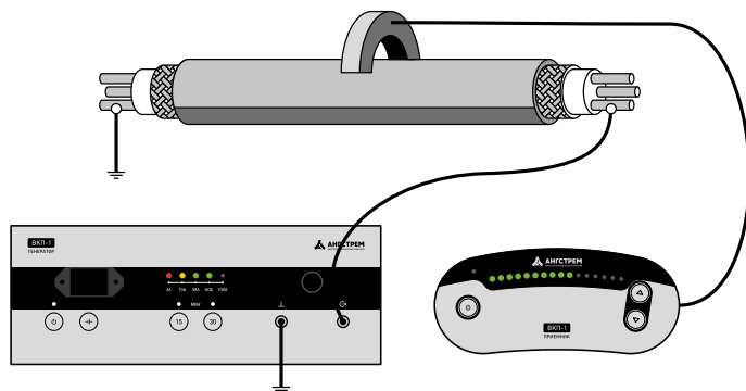
Рисунок 2 – Подключение генератора к трехфазному экранированному кабелю
