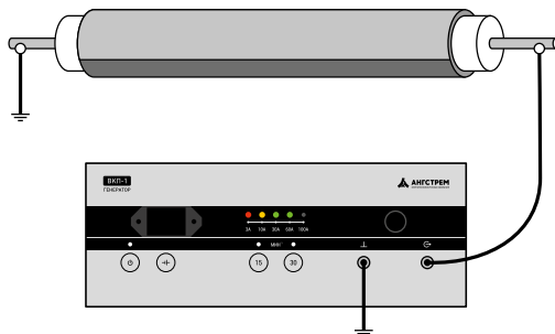
Рисунок 4 – Подключение генератора к неэкранированному кабелю
